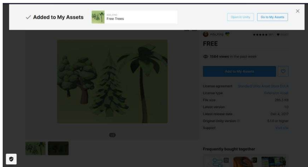
Рисунок 4.3. Добавлен ассет
