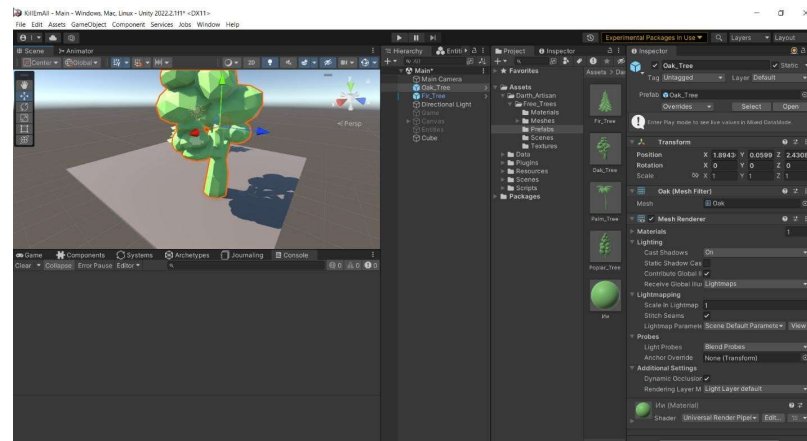
Рисунок 4.12. Настройка объекта
